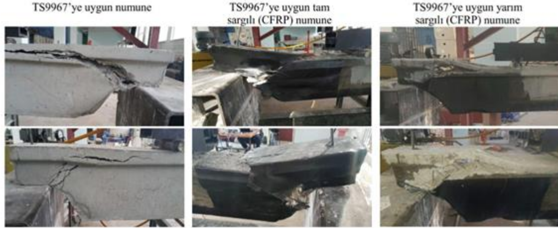
Şekil 5. İnceltilmiş uç bölgelerinde oluşan hasarlar
