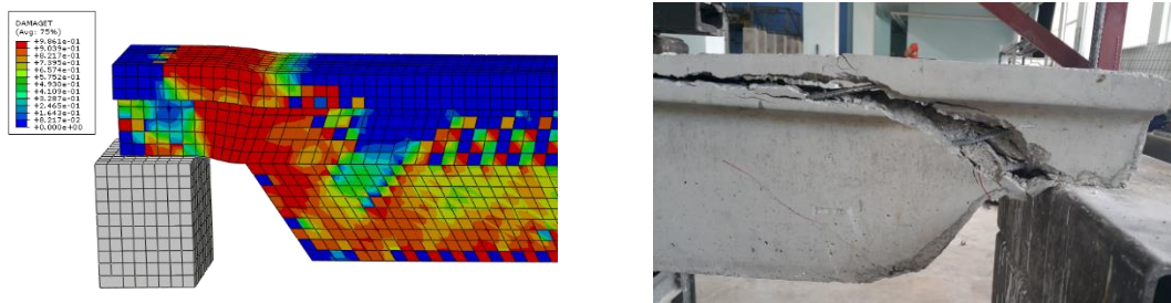
Şekil 10. TS9967'ye uygun olmayan numunelerin incetilmiş uç bölgelerinde oluşan hasarlar
