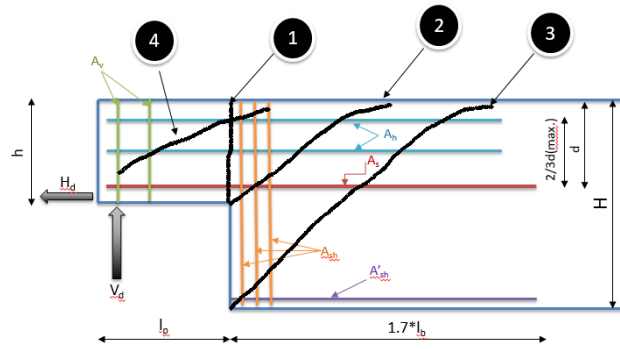
Şekil 3. TS9967'ye uygun inceltilmiş uçlu prefabrike kiriş donatı yerleşimi
