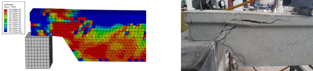
Şekil 9. TS9967'ye uygun numunelerin incetilmiş uç bölgelerinde oluşan hasarlar
