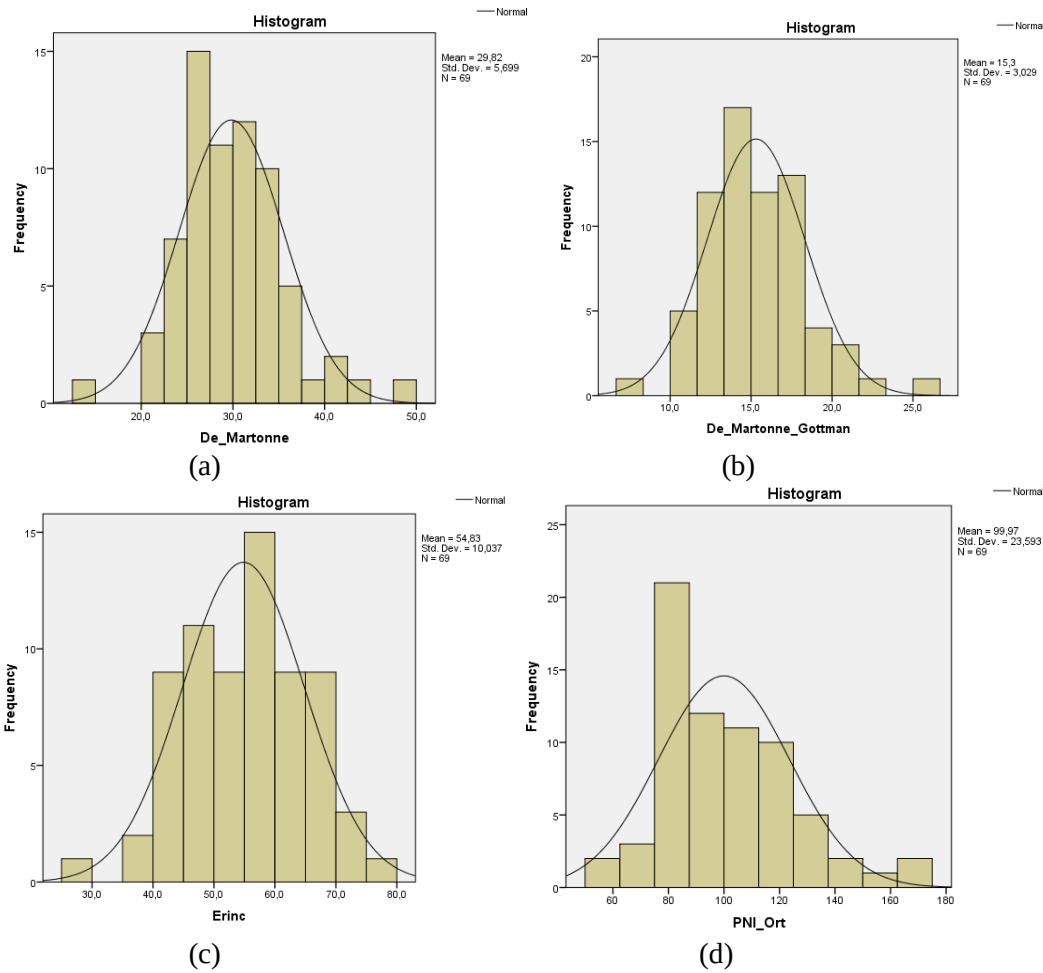
Şekil 4. Kuraklık indis değerlerinin histogram grafikleri a)De-Martonne kuraklık indis histogramı b) De-Martonne ve Gottman kuraklık indis histogramı c) Erinc indis histogramı d)PNI kuraklık indis histogramı
