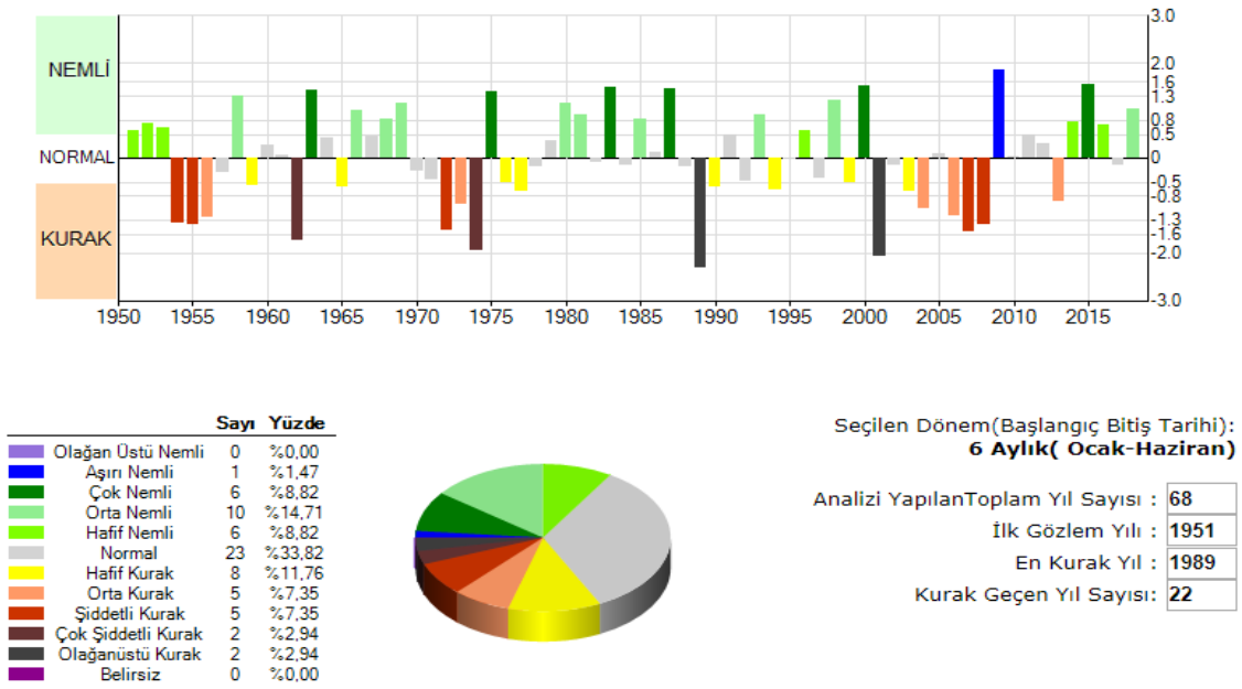
Şekil 11. Altı aylık (Ocak-Haziran) SPI kuraklık indis değerleri grafiği (URL-2)
