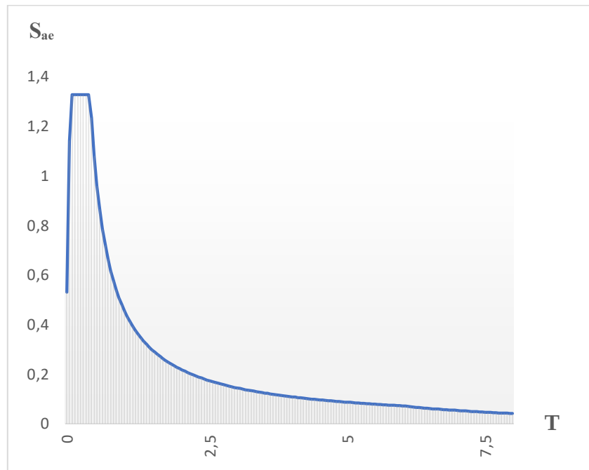
Figure 1. Lateral Elastic Design Spectrum (Afet ve Acil Durum Yönetimi Başkanlığı, 2018)
