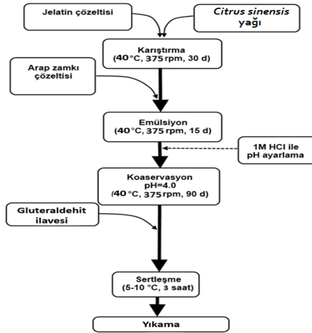
Şekil 2. Kompleks Koaservasyon Yöntemi Akış Şeması
