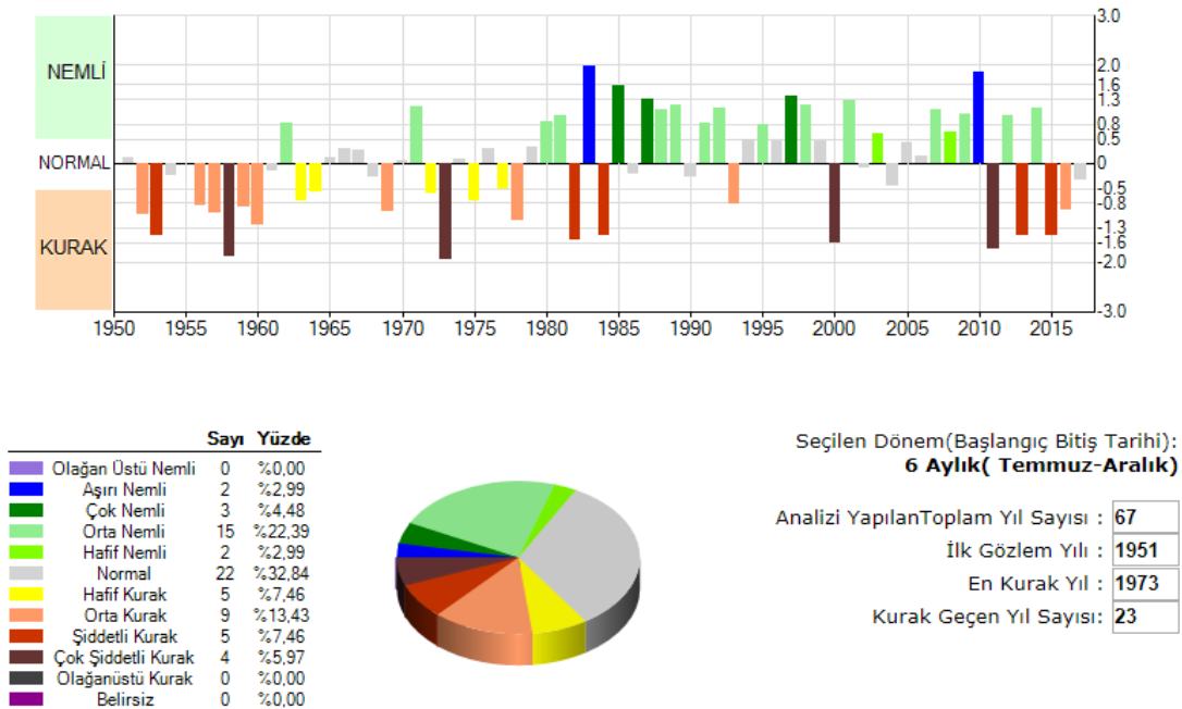
Şekil 12. Altı aylık (Temmuz-Aralık) SPI kuraklık indis değerleri grafiği (URL-2).
